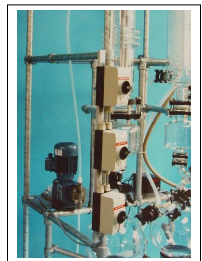
Dosierpumpe + E-Schalter
