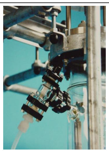
Verdampferkopf + Wischerwelle Dosierventil
